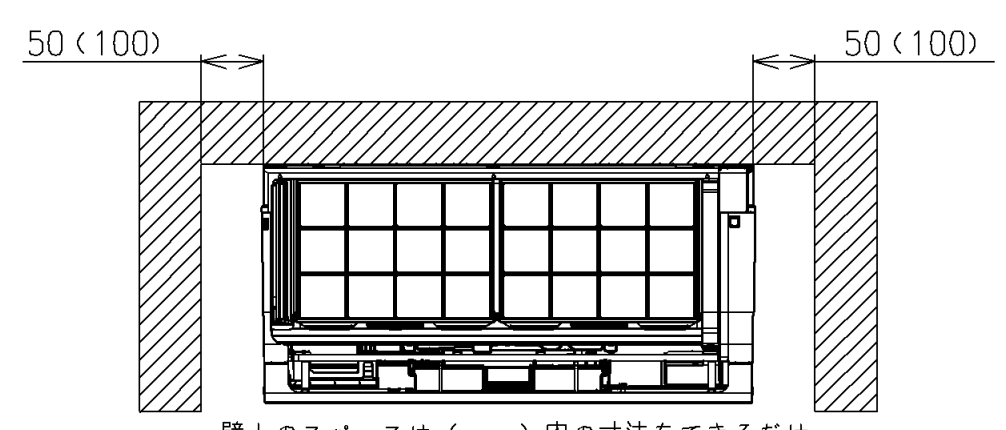
室内機サービススペース
