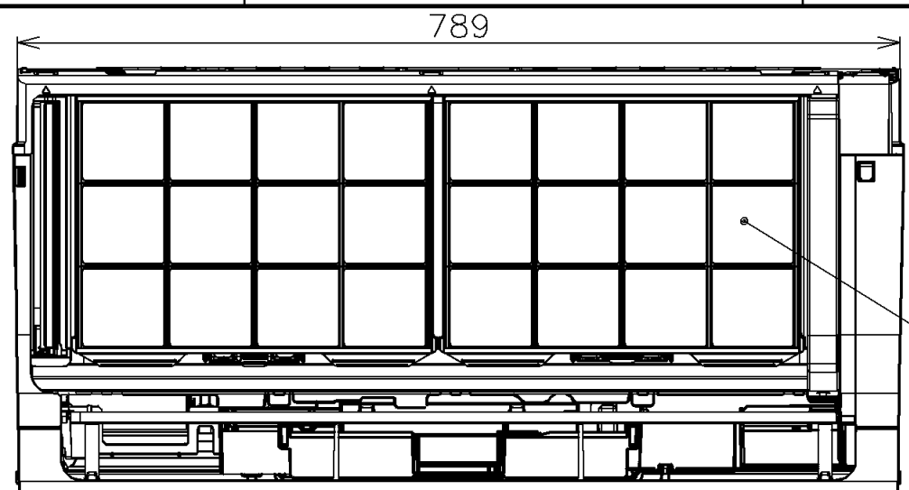
日立ルームエアコン壁掛ZJシリーズ 室内ユニット寸法図
